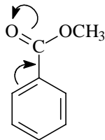
Esters
