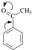
Ketones
